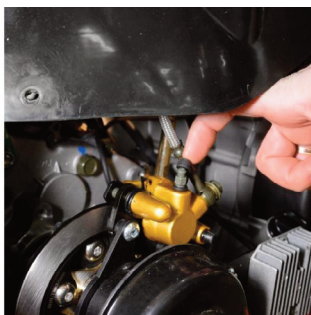
ВИНТ КЛАПАНА ВЫПУСКА ВОЗДУХА
